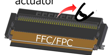
STEP 2. Close actuator
